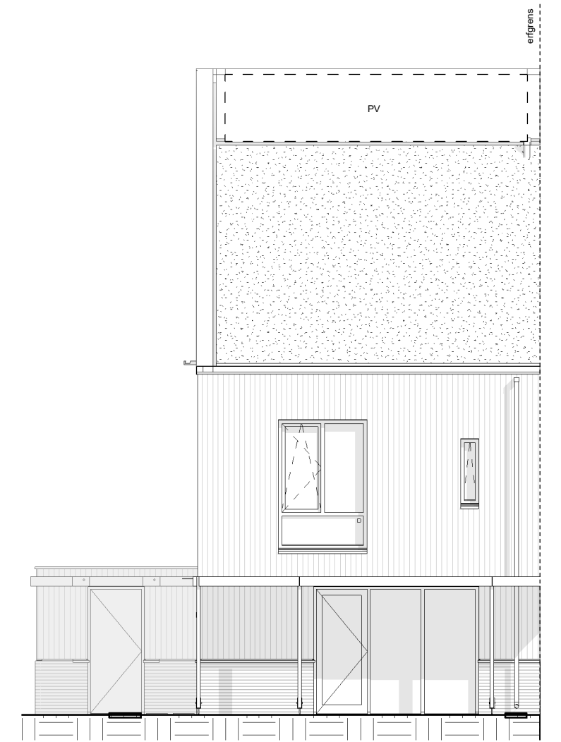
voorgevel (oost)
