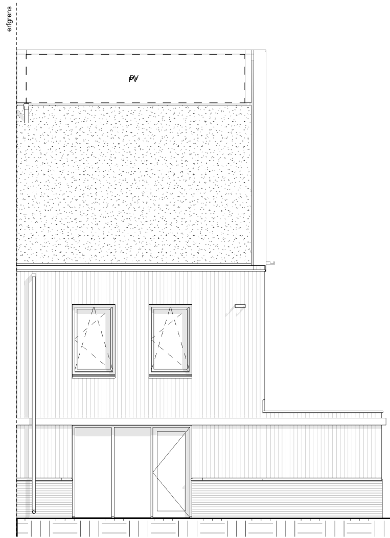
achtergevel (west)
